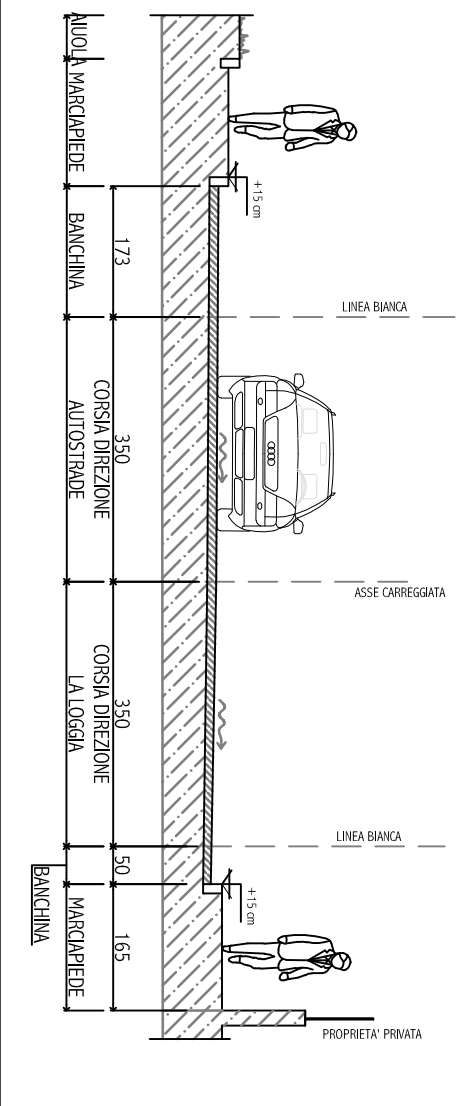
SEZIONE E-E - Scala 1:100
